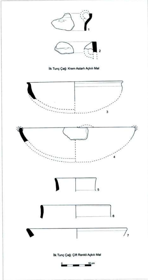
Çizim 13: İlk Tunç Çağ Çanak Çömleđi
