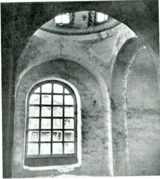
Res. 21 — Paraklesiyon üzerindeki galeri. Fig. 21 — The gallery above the Parecclesion.
