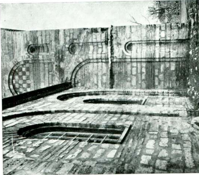
Res. 25 — Dış galerilerin paraklesiyondan daha sonra yapılmış bir ek olduğuna şüphe bırakmayan mimarî bir vesika ve inşâî teknik. Fig. 25 — Walls, the structure of which proves that the outer galleries have been built at a later date than the parecclesion.
