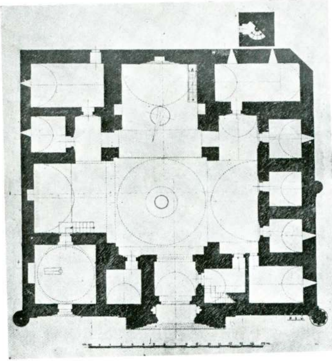
Res. 1 — Caca bey Medresesi'nin genel plânı. (Bk. A. Saim Ülgen, Vakıflar Dergisi, sayı 2, s. 261, Res. 1).
