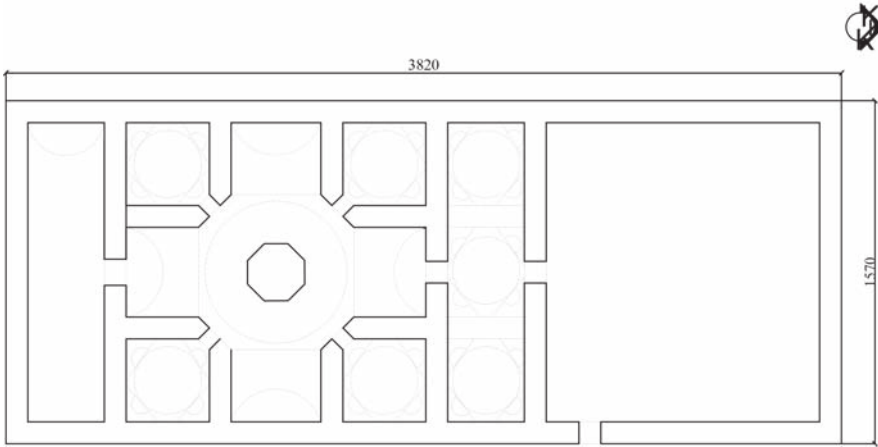
Çizim 4. Taşçı hamamı planı.
