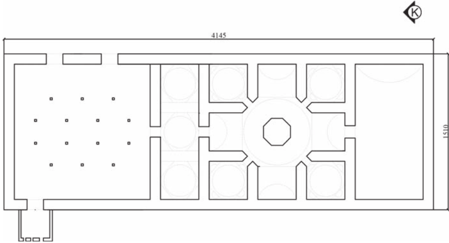
Çizim 2. İzzet Paşa hamamı planı.
