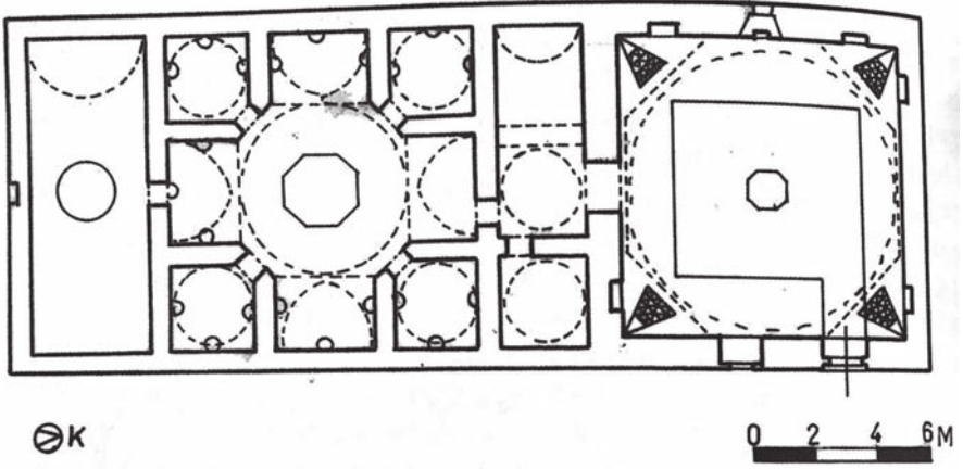
Çizim 1. Çadırçı hamamı planı (H.Özkan'dan).
