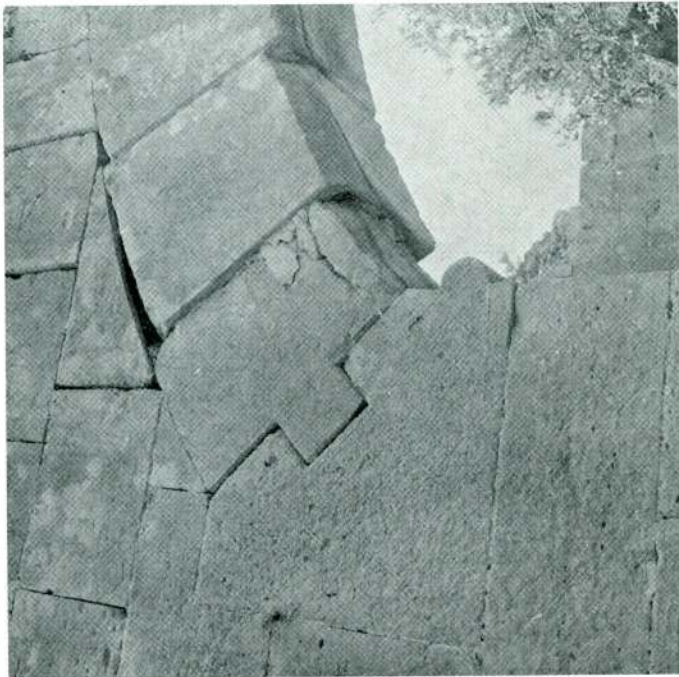
8 — Dış portalin kemer başlangıcı detayı Detail of the arch of the main portal. ( Tükel arşivi neg. no. 60882 .)
