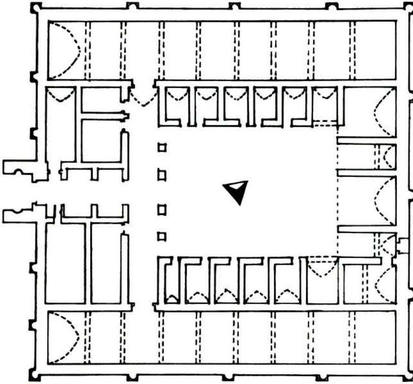
22 — Tercan Mama Hatun Kervansarayı - plan rölevesi (Vakıflar Genel Müdürlüğü) Tercan Mama Hatun Caravanserai - plan
