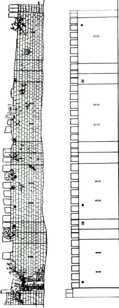
5 — a) Batı cephe (şimdiği hali) West elevation - actual b) Batı cephe - restitüsyon West elevation - reconstruction
