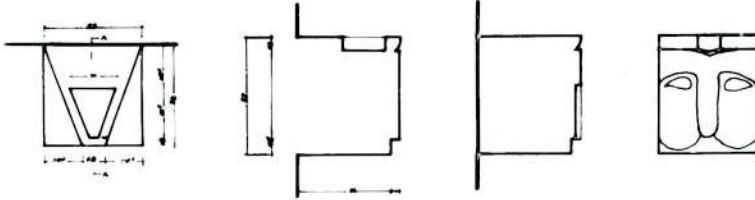
17 — Arslan başı kandilliklerinin üst görünüş, kesit, yan ve ön görünüşü. The top view section, Side and front elevations the candle brackets.
