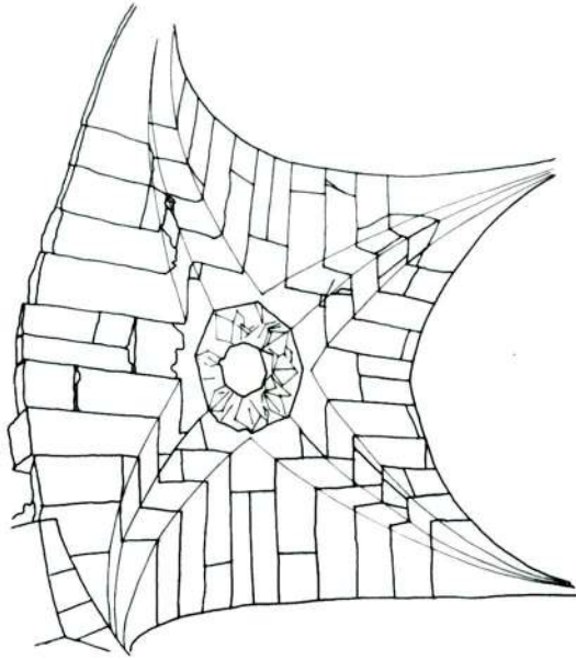
15 — Yıldız tonozun çeşitli detayları Various details of the star vault.
