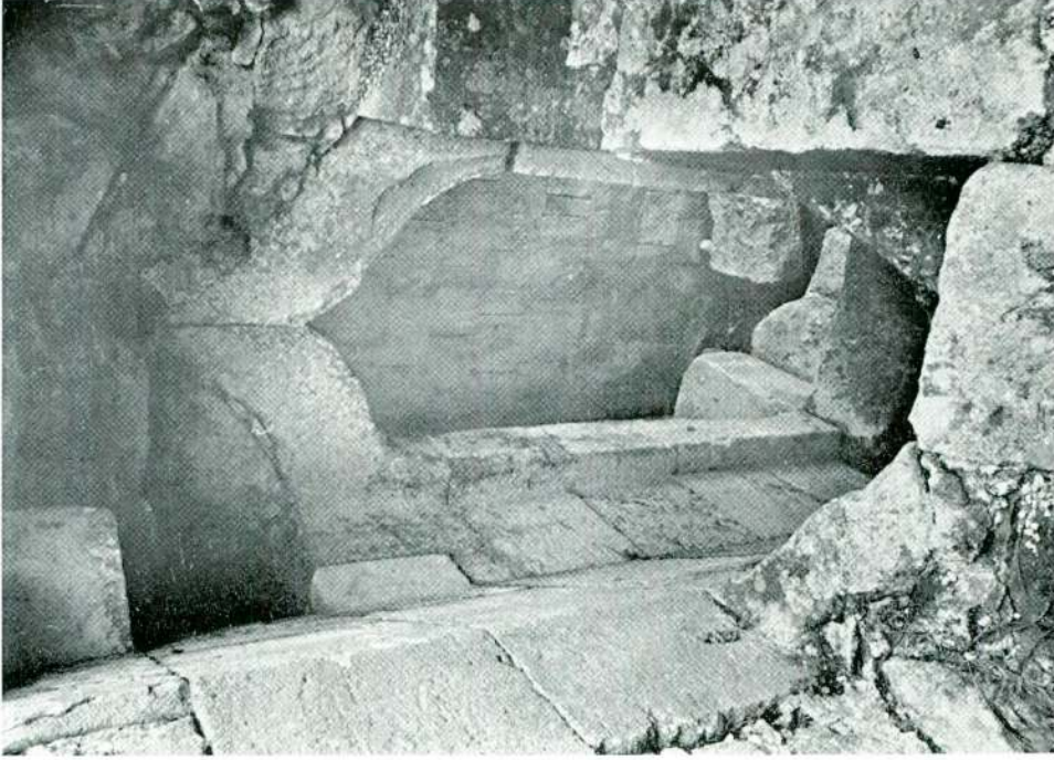
15 — Merdivenin dogu payanda içinde dönerek devam eden kısmı. The winding part of the stairs within the east abutment ( Tükel arşivi neg. no. 35/198 )
