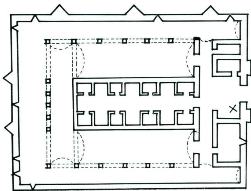
18 — Alara Han plân rölevesi (F. Erten) Alara Han plan (F. Erten)
