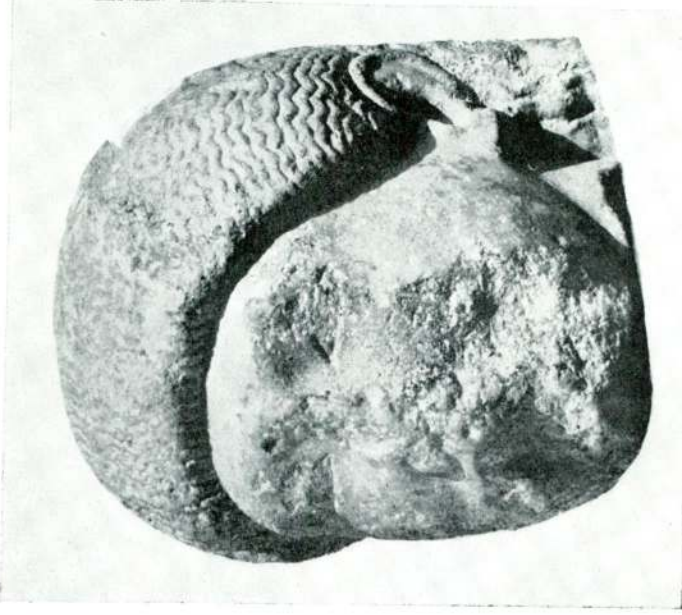
Res. 2 — İzmit Kuros'unun dördte üç cepheden görünüşü.
