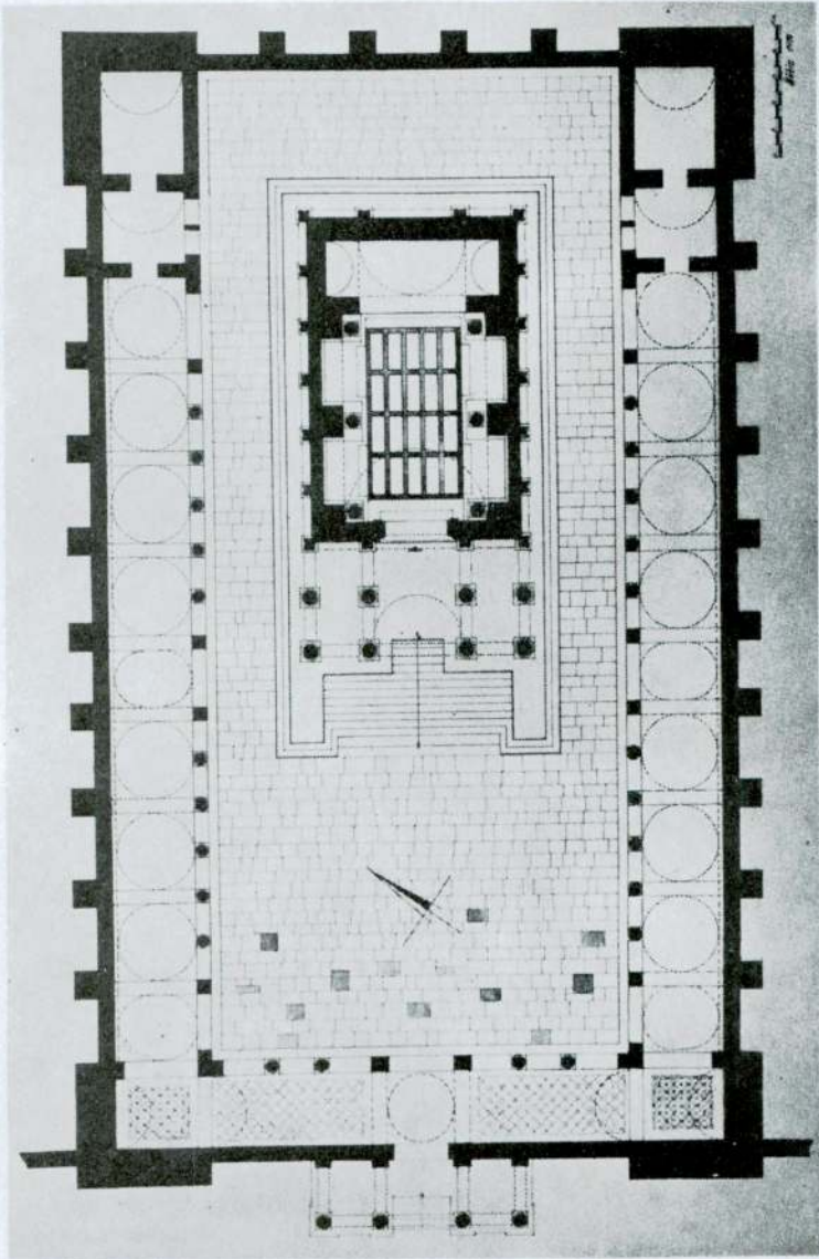
Res. 8 — Side, Batı Mavsoleumu'nun plânı.
