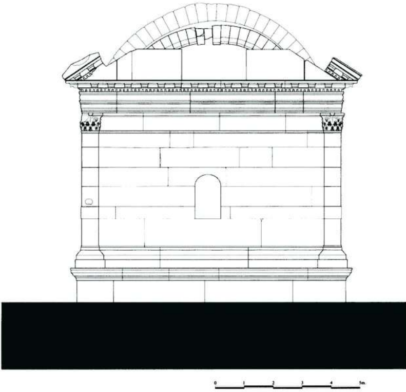
Çizim 3 - Anıtın Arka-Kuzeydoğu Cephesi Rölövesi
