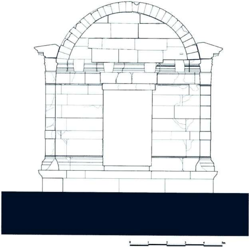
Çizim 2 - Anıtın Ön-Güneybatı Cephesi Rölövesi
