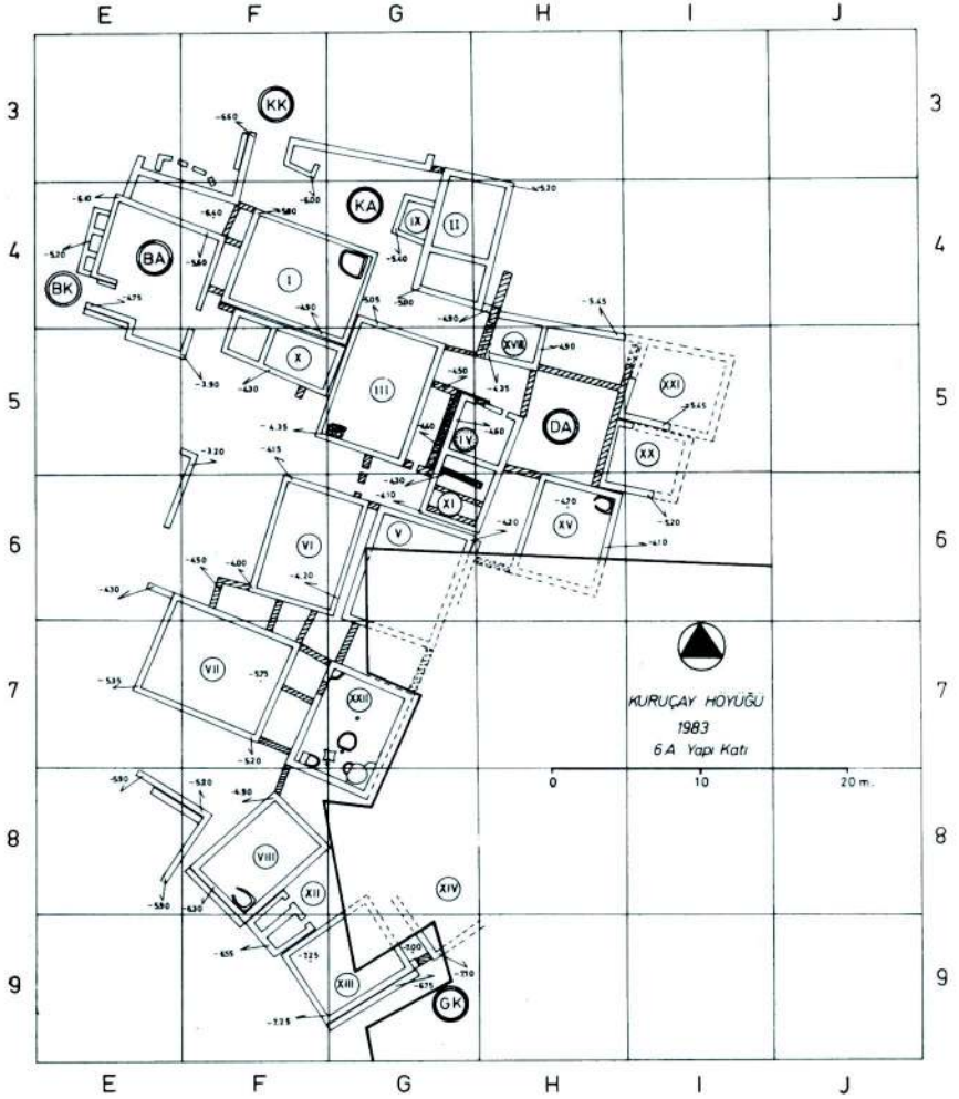
Res. 7 — 6 A Yapı Katı planı (Taramalı duvarlar 6 A 1 evresine aittir
