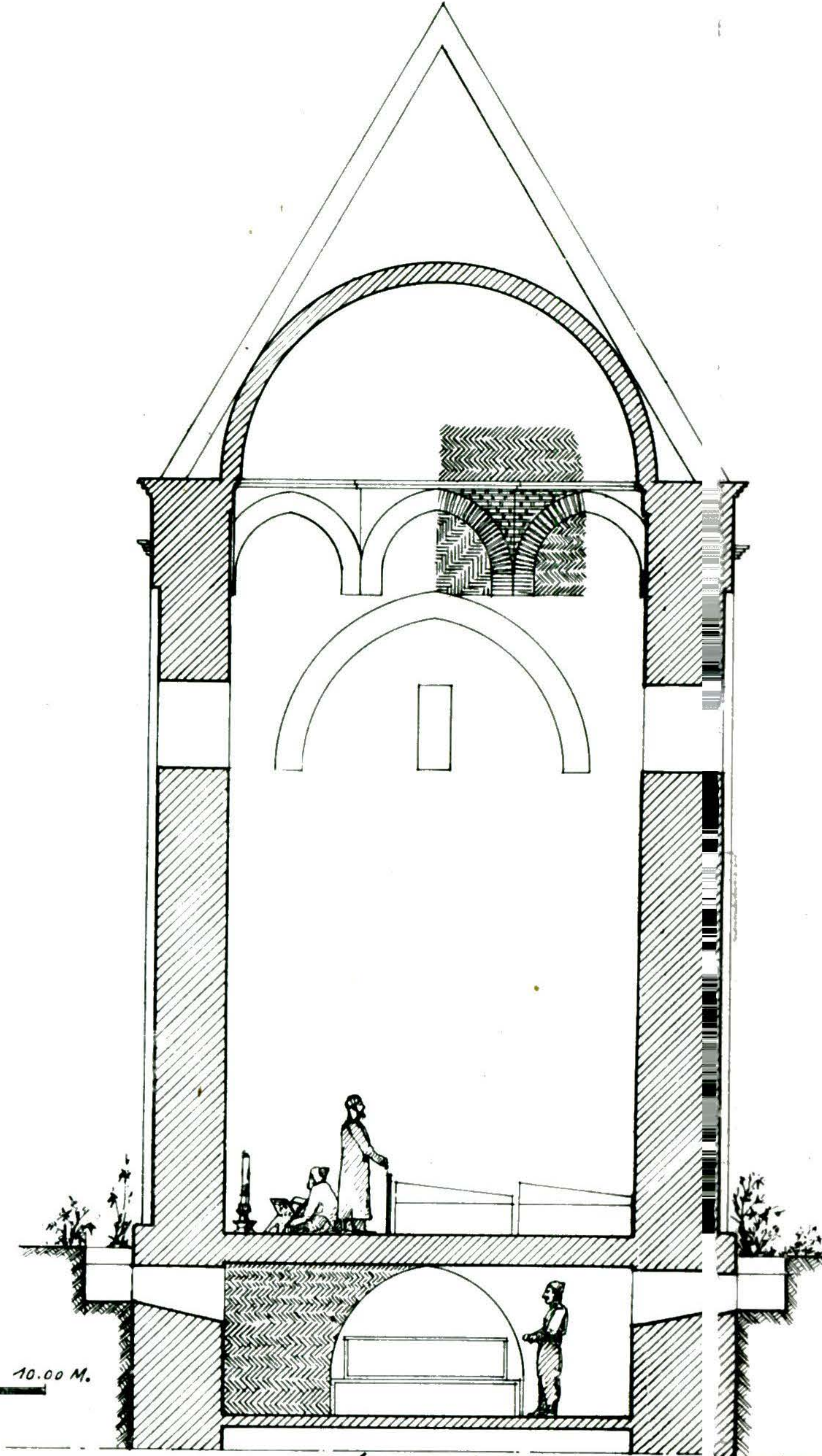
A, A KESİTİ
