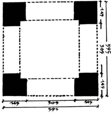
Res. 6 — Kubadiye'deki bina kalıntısının plânı.
