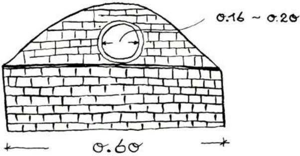
Res. 2 — Kubadiye Saraylarına su getiren Künklerin duvar içindeki durumu.
