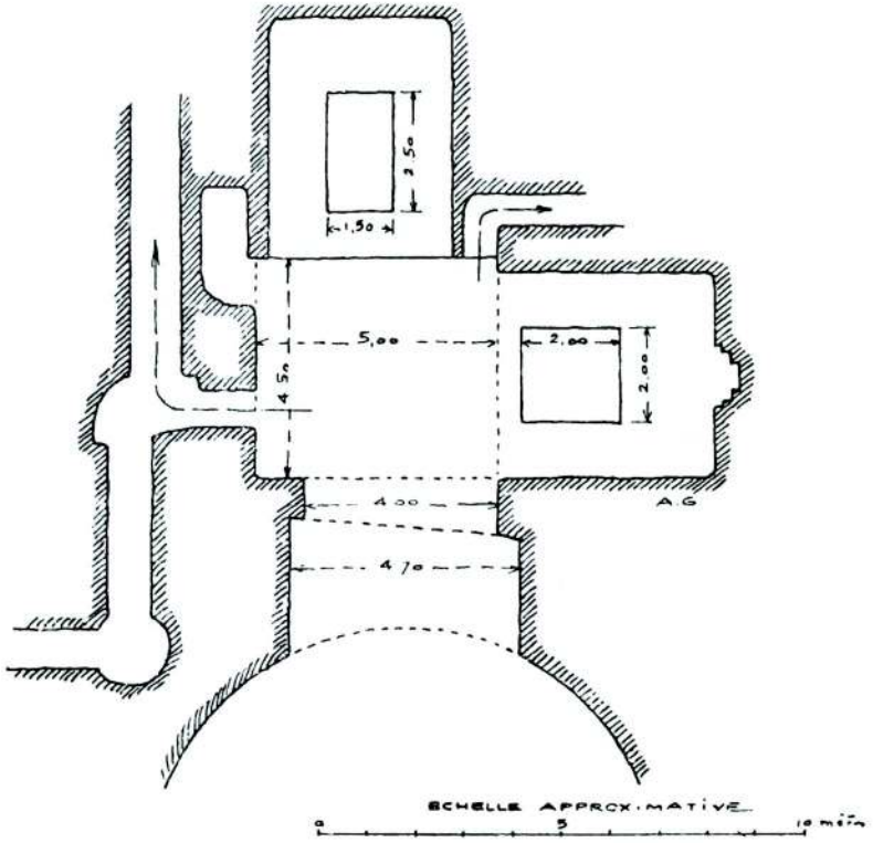
FIG. 12. — PLAN DES CROITÉS
