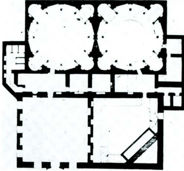
Res. 15 — Çemberlitaş'da Valide Sultan Hamamı plânı (H. Glück)
