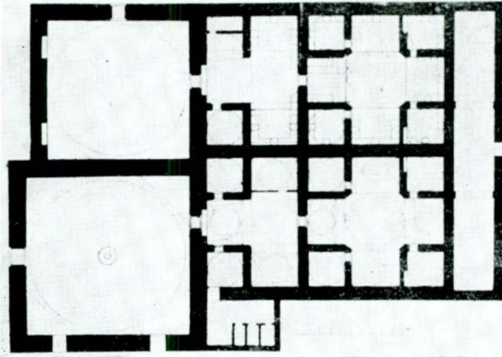
Res. 10 — Bayezid Hamamı plânı (H. Glück)
