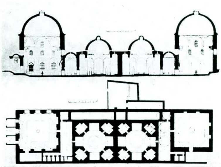
Res. 11 — Ayasofya da Hamâm-ı Sultânî. Mimar Koca Sinan eseri (H. Glück)
