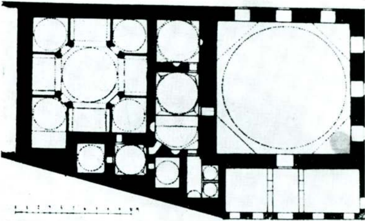
Res. 12 — Mimar Koca Sinan yapısı Süleymaniye Hamamı plânı (H. Glück)
