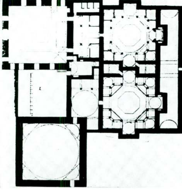
Res. 13 — Cağaloğlu Hamamı plâni (H. Glück)
