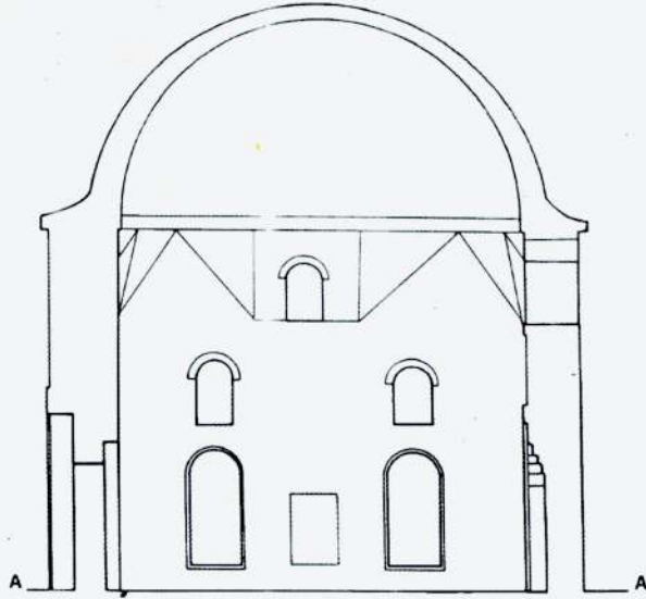
Şekil 2. Edirne- Karaağaç Timurtas Köyü Timurtas Paşa Camisi'nin A- A kesiti
