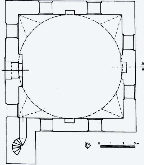
Şekil 1. Edirne- Karaağaç Timurtas Köyü Timurtas Paşa Camisi'nin planı
