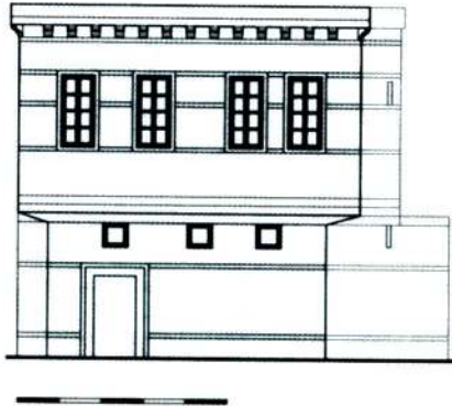
Şekil 11 - 5 No'lu örneğe ait zemin - birinci kat planı ve ön görünüş (Avni Bey'in evi)
