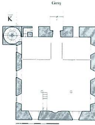
Şekil 6 - Camii planı
