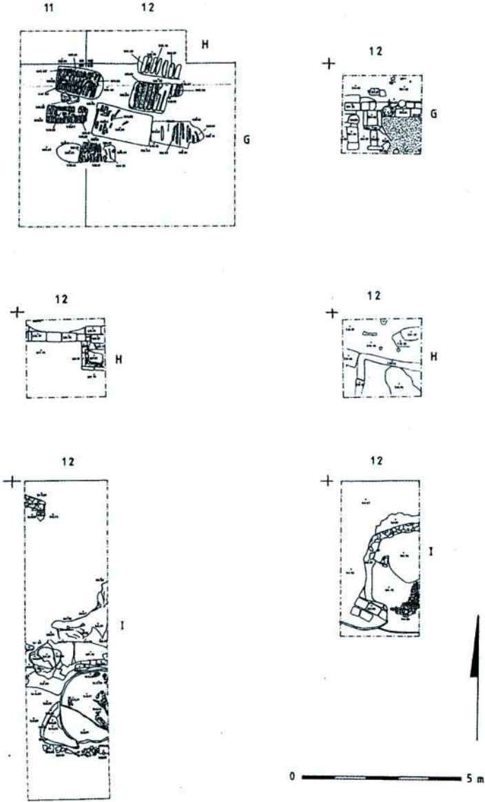
Çizim 5 - G 12, H 12 ve I 12 Açma Planları
