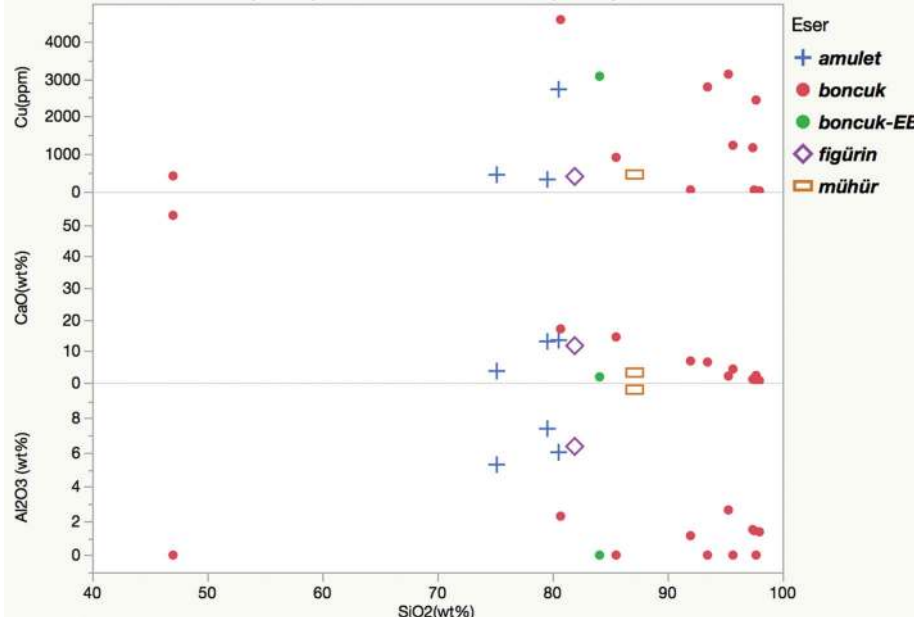
Resim 12: Acemhöyük vitrifiye buluntularında, silika (SiO 2 , wt%) oranlarının alüminyum oksit (Al 2 O 3 , wt%), kalsiyum oksit (CaO, wt%) ve bakır (Cu, ppm) oranlarına göre dağılım grafikleri. Grafiklerde figürin, amulet ve mühürün boncuklardan çoğunlukla ayrı gruplanması dikkat çekicidir.
