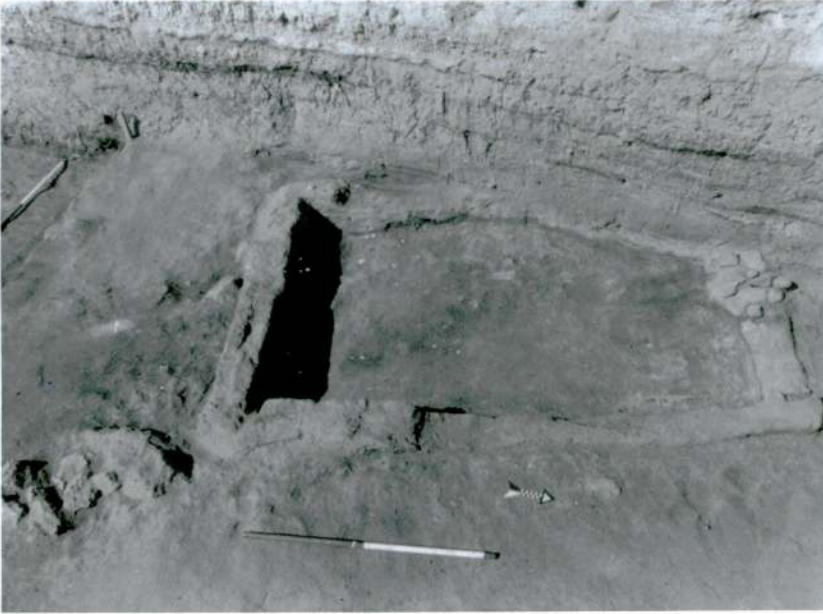
Levha 4/2 - ENÇ 4 katı yapısı
