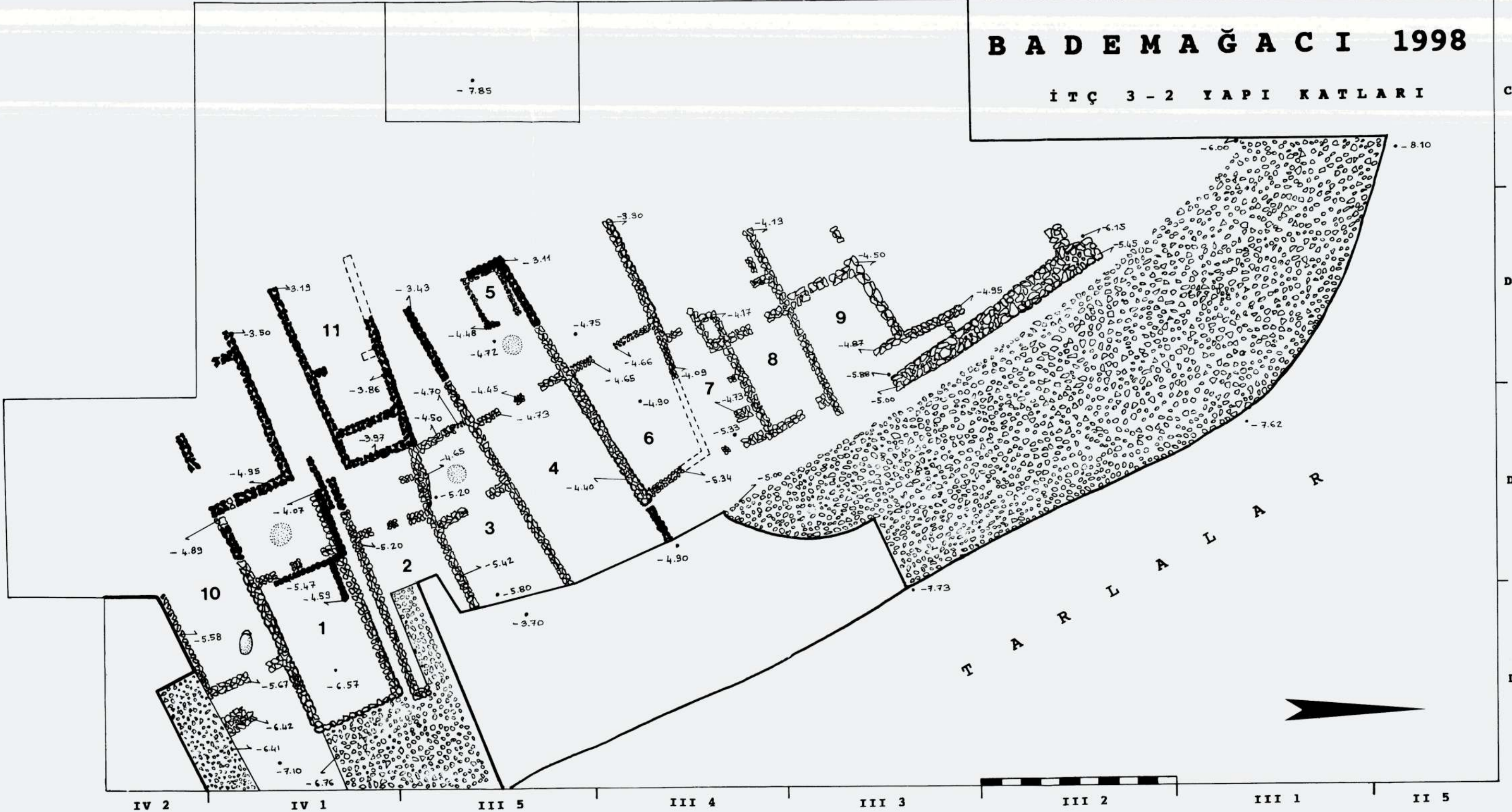
Levha 18 - İTÇ 3-2 yapı katları planı
