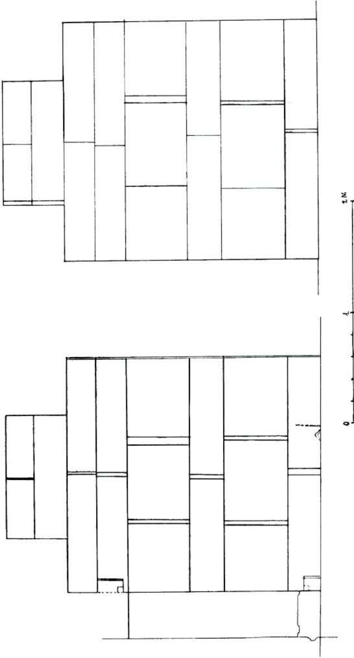
Res. 7 — Mezar odasının iç duvar rölevelederi. Sağda batı, solda güney tarafı (S. Kasper)
