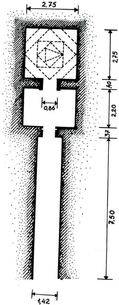
Res. 18 — Musahocaköy mezarının plan krokisi (N. Firath)
