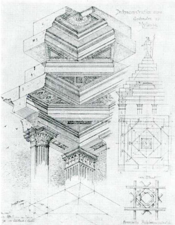
Res. 20 — Milas "Gümüşkesen" mezarının tavan konstrüksiyonu (J. Durm)
