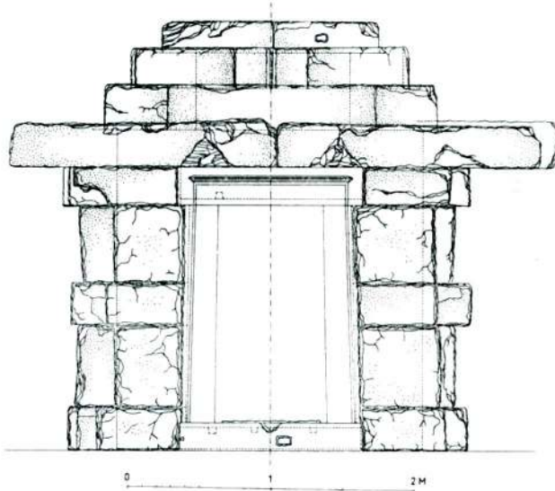
Res. 8 — Mezar odasının dođu cephesi (a) ve rölevesi (b) (S. Kasper)
