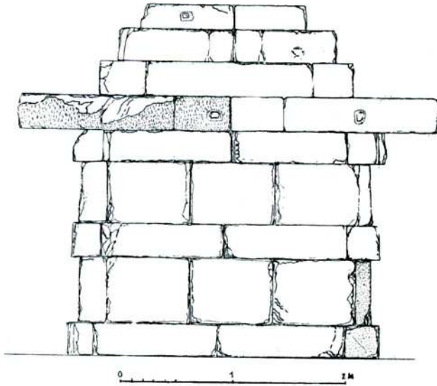
Res. 11 — Mezar odasının batı tarafı (a) ve rölevesi (b) (S. Kasper)
