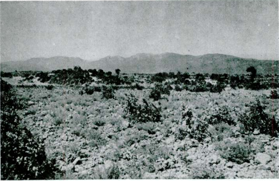
(res. 25)— Leçe kesimindeki bazalt sivrintileri (batdan bakış). (Abb. 25)— Die Basaltrücken im Abschnitt von Leçe von Westen gesehen.
