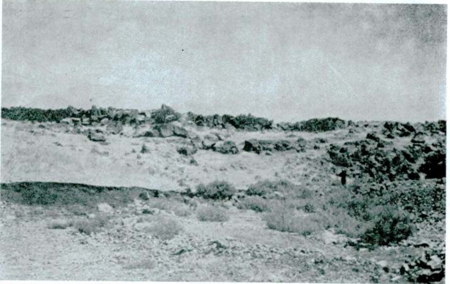
(res. 28)— Bađlama kesimindeki bazalt sivrintilerinin gneyden diđer' bir grnř. (Abb. 28)— Die Basaltrcken im Abschnitt von Bađlama, eine andere Ansicht.
